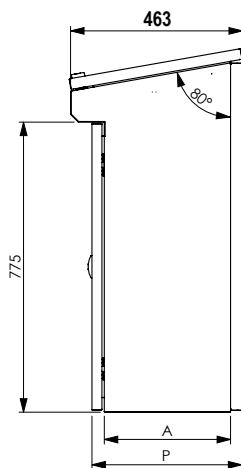
Vista laterale
